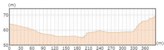
C-D断面図
